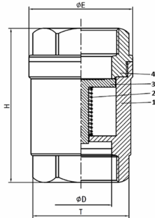
Dimensiones en (mm.) / Dimensions in (mm.)
